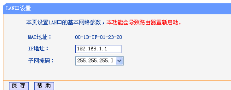
图 5-9 LAN 口设置
